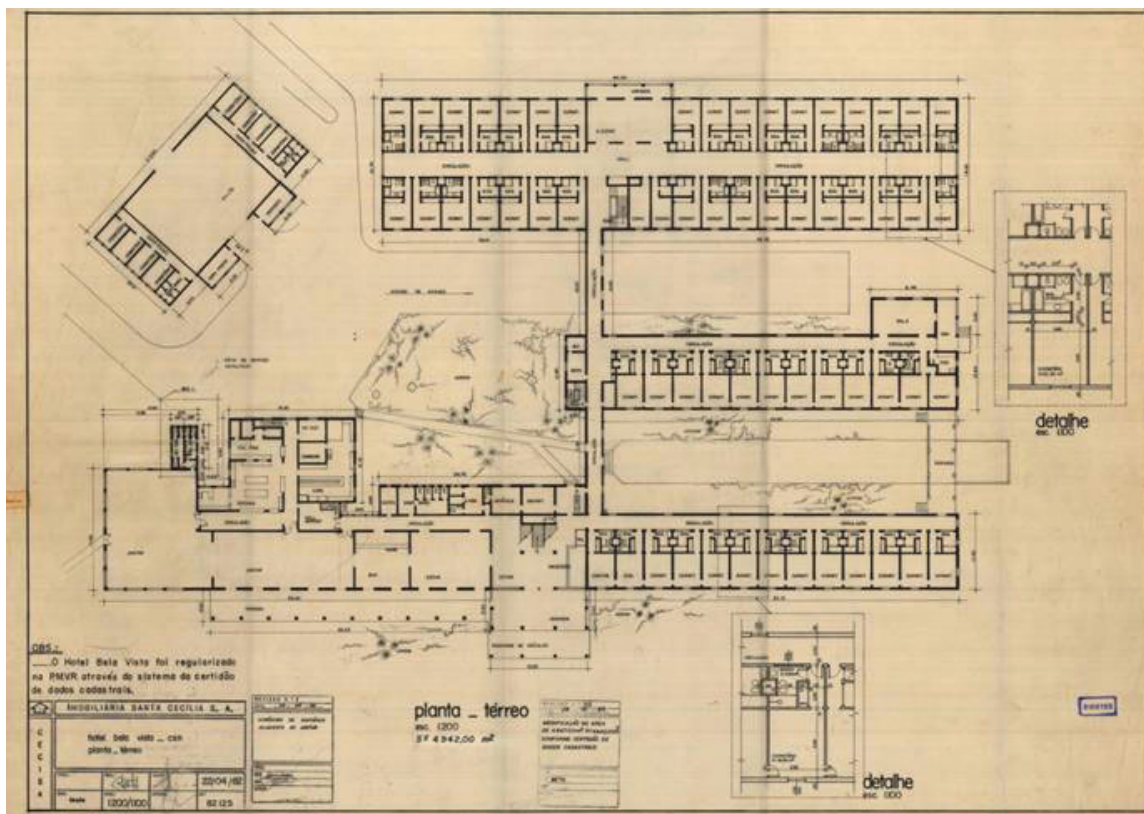
Figura 19 – Projeto Construtivo – Pavimento Têrreo (1982).
