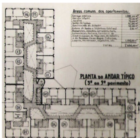
Figura 5 - Planta Baixa dos apartamentos
